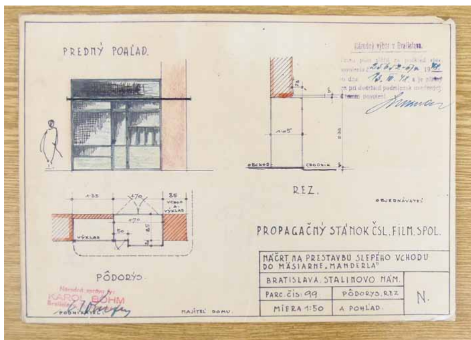
12. PÔDORYS A POHĽAD PROPAGAČNÉHO STÄNKU
