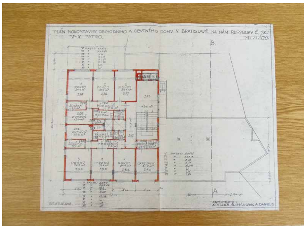
6. MANDERLA, PÔDORYS POSCHODÍ VI-X.
