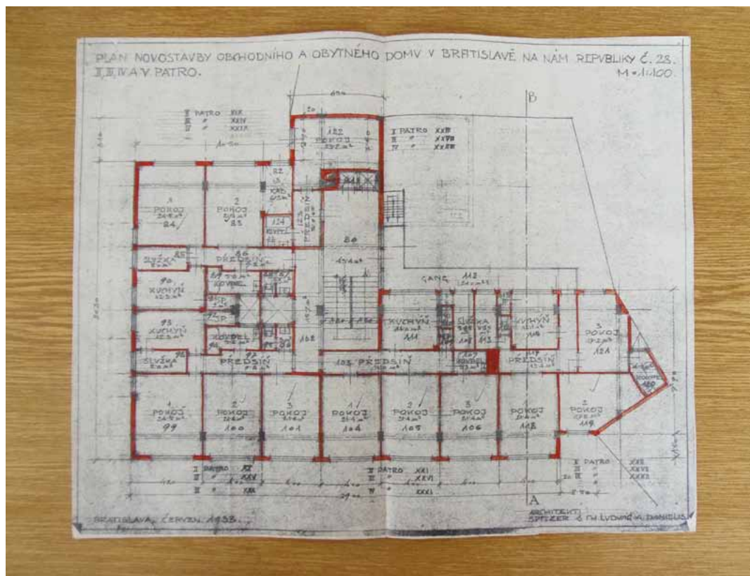
5. MANDERLA, PÔDORYS POSCHODÍ I-V.
