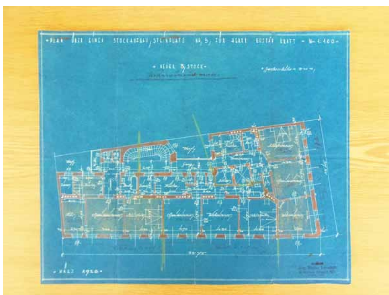
15. PÔDORYS JEDNOPOSCHODOVÉHO DOMU, KAMENNÉ NÁMESTIE 5, 1929
