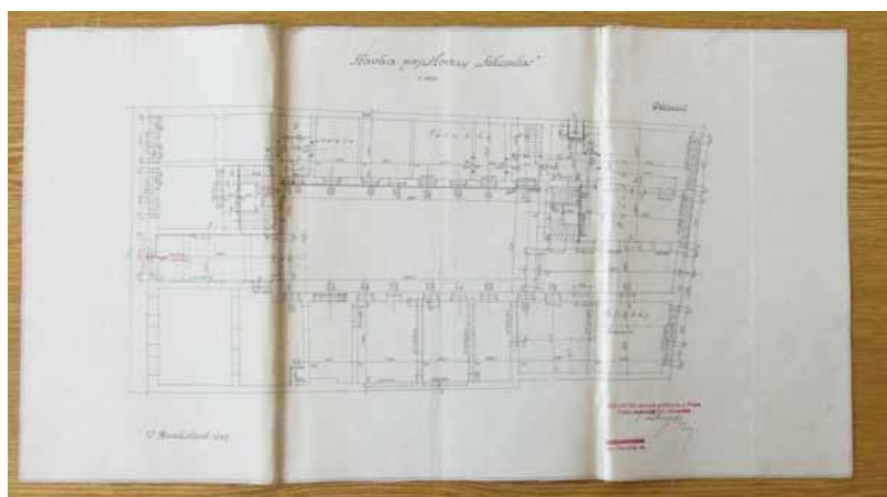
14. PÔDORYS BUDOVY POIŠŤOVNE SECURITAS, 1929
